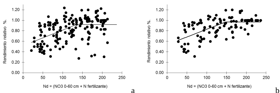
Figura 2. Rendimiento relativo del cultivo de colza en función del nitrógeno disponible (N disponible (Nd): N de nitratos en suelo hasta 60 cm + N de fertilizante, aplicado al estadio de roseta). a) Respuesta al agregado de N sin aporte de S b) Respuesta al agregado de N con aporte de S.
