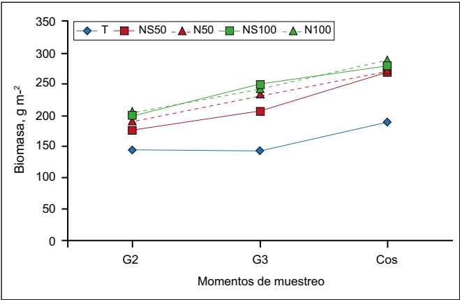
Figura 2. Evolución de la biomasa (g m 2 ) en los diferentes tratamientos de fertilización en colza. Campaña 2016. Villa Elisa, Entre Ríos.
