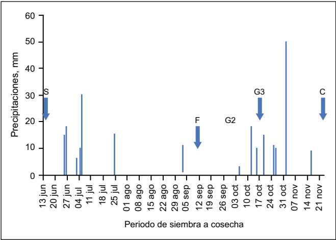
Figura 1. Precipitaciones (mm) desde siembra a cosecha. Las flechas indican distintos estados fenológicos S (siembra), F (floración), G2 (silicuas menores a 4 cm), G3 (silicuas de 4 cm) y C (cosecha). Campaña 2016. Villa Elisa, Entre Ríos.
